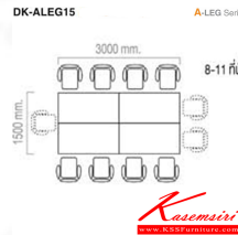
DK-ALEG15 โต๊ะ: ขา A-LEG 1500(W) x 750(D) x 750(H) mm.
