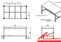
SPD-150NB เกรด 304 ทังตัว W150xD80xH64 CM.
