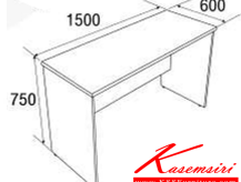
2EXCF615 โต๊ะต่อโต๊ะประชุม 1500(W) x 600(D) x 750(H) mm.
