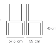
PN92154 Dim. 57.5 x 55 x 73 cm
