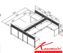
Modular MT-WS024 (ชุด workstation 4 ที่นั่ง) 3310(W) x 3255(D) x 1200(H) mm.
