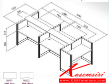
MT-WA014R (TOP ตรง) / MT-WA024R (TOP Wave) 3183(W) x 1255(D) x 1083(H) mm. (ชุด workstation 5 ที่นั่ง) จุดเด่น : เพิ่มเต็มพื้นที่ใช้งาน แบบเดี่ยว 1 ที่นั่ง บริเวณหัวหรือท้ายชุด
