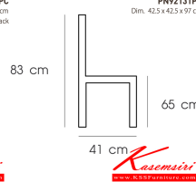
PN92131PC Dim. 42.5 x 42.5 x 97 cm
