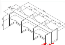
MT-WA016 (TOP ตรง) / MT-WA026 (TOP Wave) 3860(W) x 1255(D) x 1083(H) mm. (ชุด workstation 6 ที่นั่ง)
