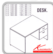
ท็อปไม้หนา 25 มม. ปิด EdgePVC 1 มม. แผ่นข้างหนา 19 มม. ปิด EdgePVC 1 มม. แผ่นนั่งตาหนา 16 มม. ปิด EdgePVC 0.5 มม.
