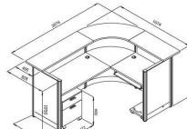
2CT120 ชุดเคาน์เตอร์ประชาสัมพันธ์ L-shape 2074(W) x 1674(D) x 1083(H) mm.
